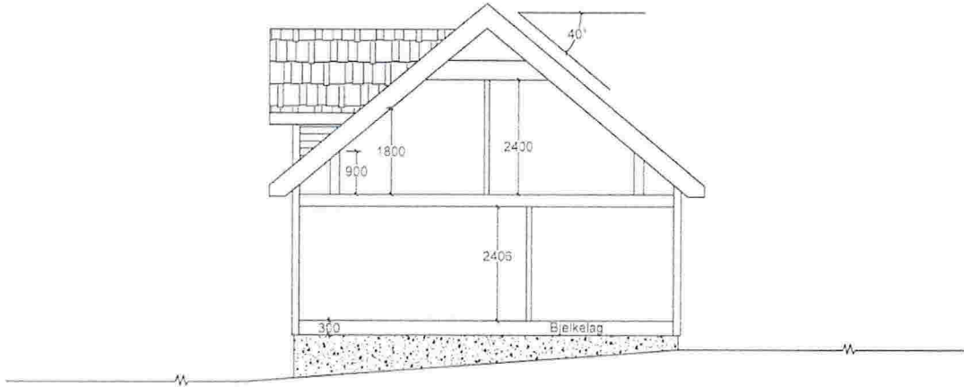
Snitt sett mot nordvest
