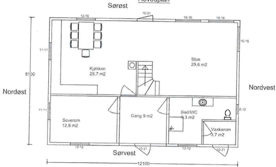
Hovedplan
