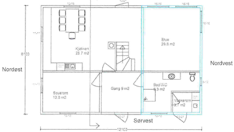
Hovedplan Sørøst
