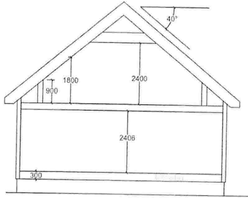
Snitt sett mot nordvest
