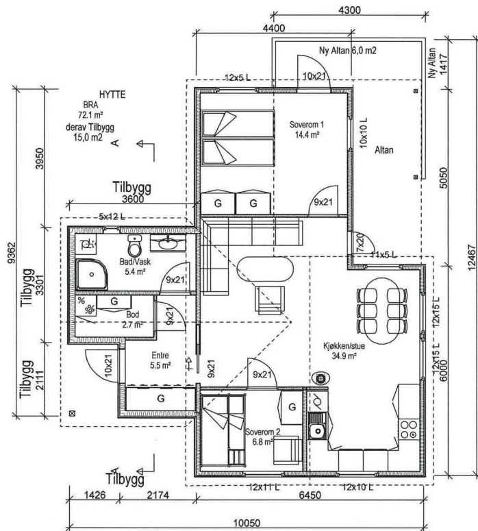
Hovedplan
