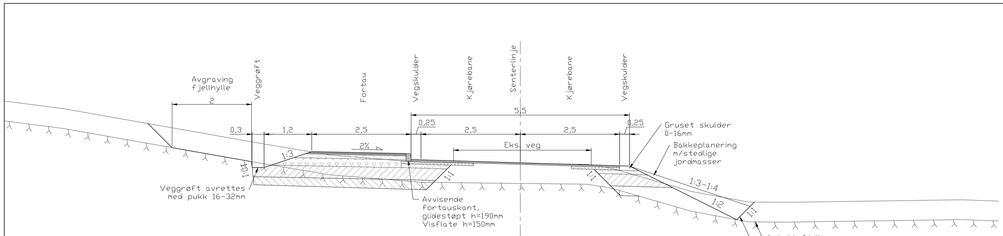
NORMALPROFIL Fv391 - LEIKNESVEGEN Veg o_V M=1:50
