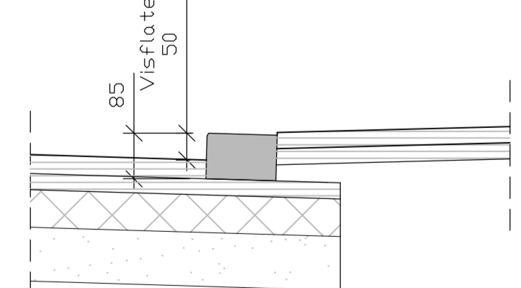
NEDSENKET FORTAUSKANT I AVKJØRSLER M=1:10
