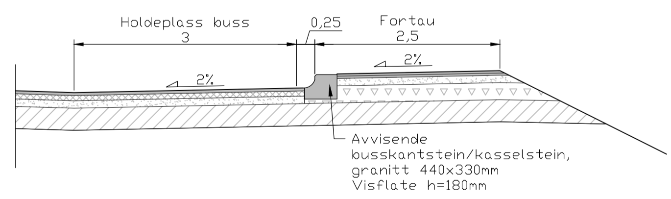
SNITT BUSSHOLDEPlass M=1:50 Lengde=20m Utvidelse og innsnevring over 15m
