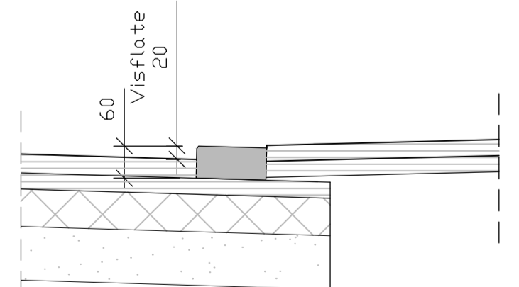
NEDSENKET FORTAUSKANT I KRYSNINGSPUNKT FOR FOTJENGERE M=1:10
