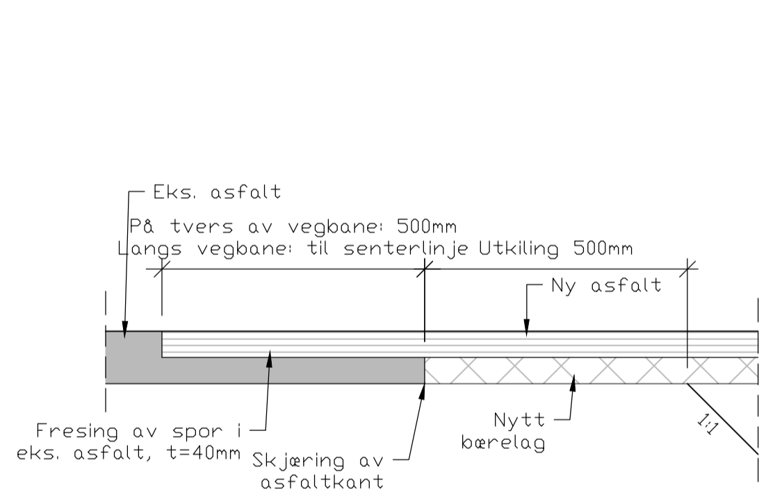
OVERGANG EKISTERENDE/ NY ASFALT M=1:10
