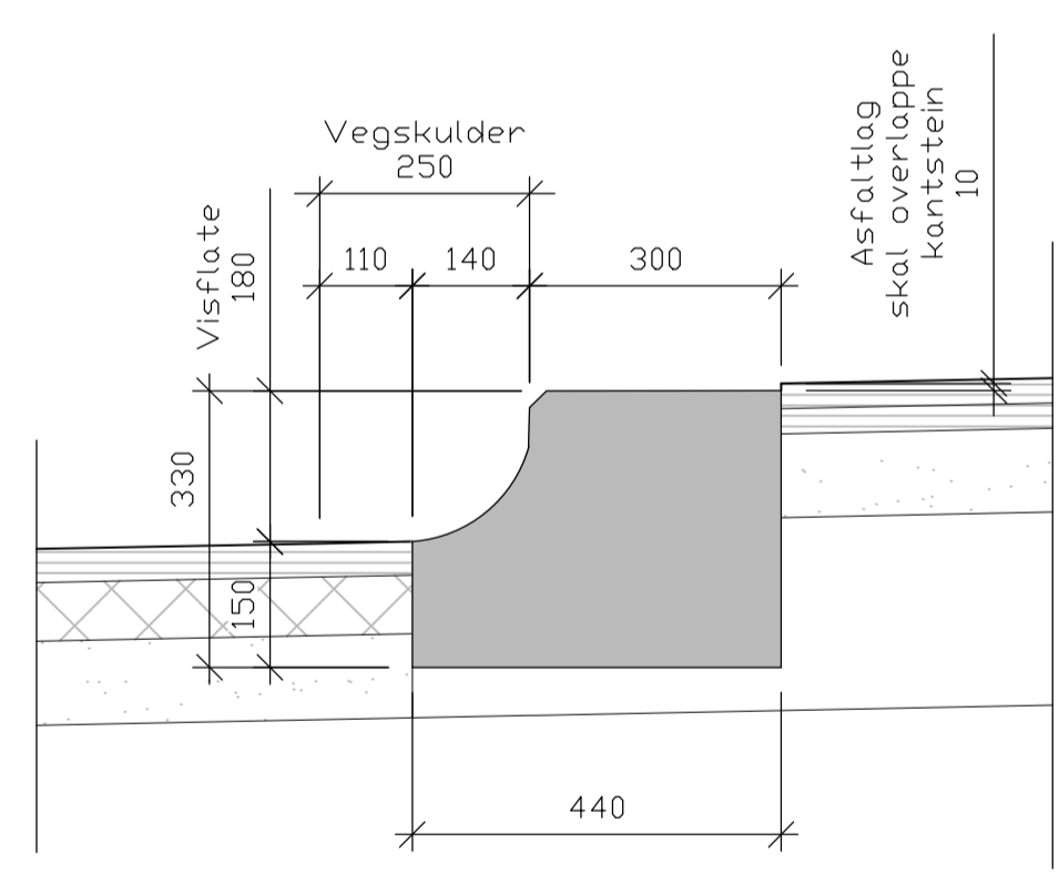
AVSLUTNING ASFALT MOT KASSELKANTSTEIN M=1:10
