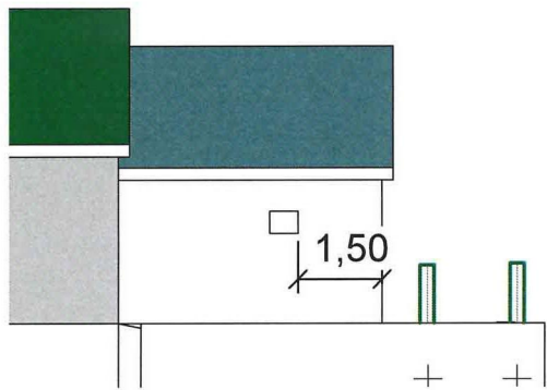
③ Section 11 1 : 100
