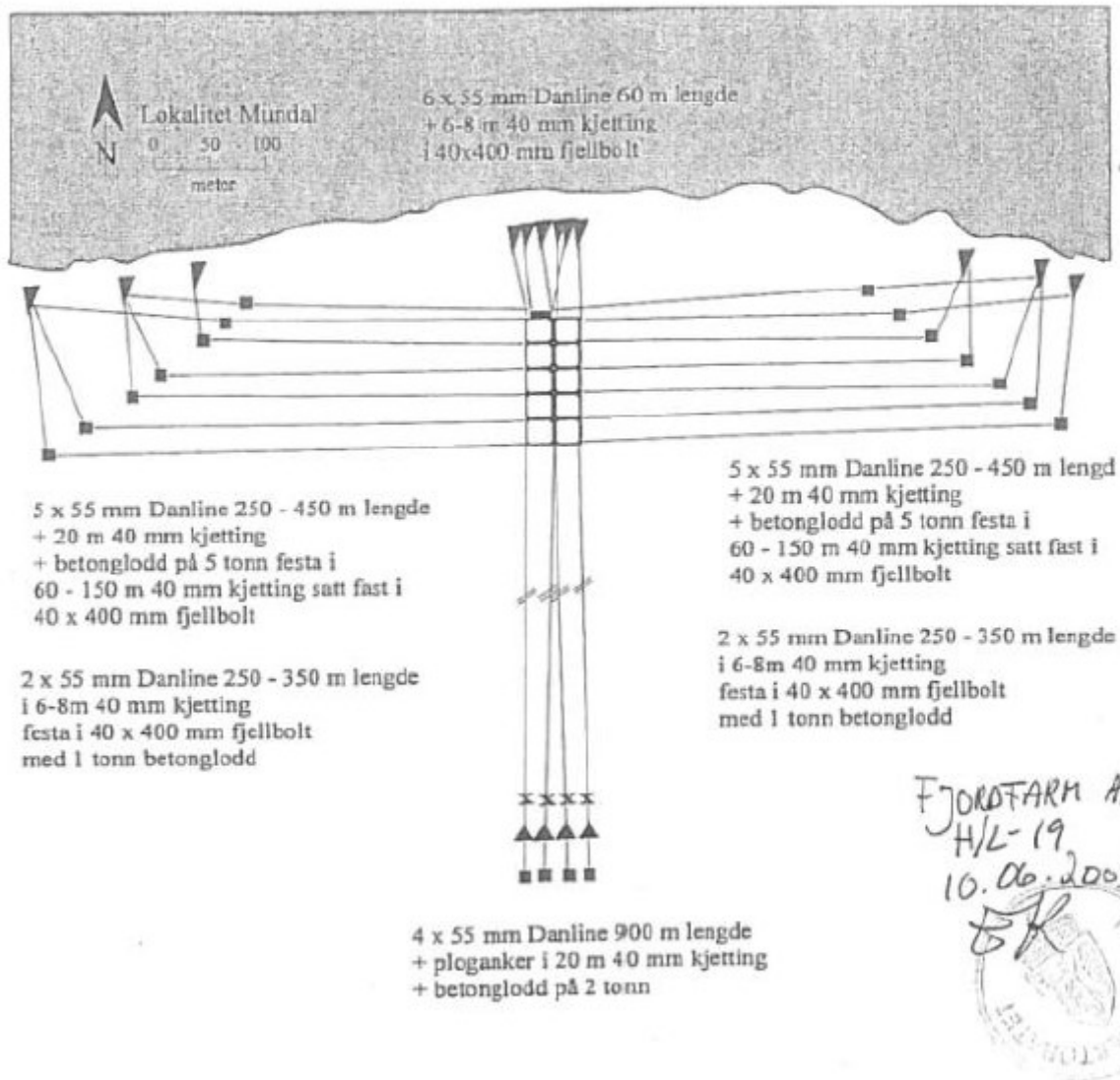
Figur 4.3. Plassering av anlegget med fortøyningsplan ca 90 m frå land ved Mundal teikna etter økonomisk kartverk (M= 1:5 000). Kartreferanse, sjokart: N 60°33,82' E 05°21,54'.
