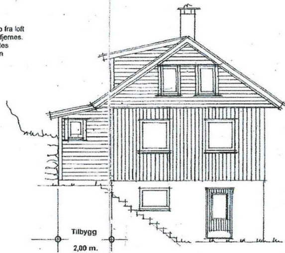
Fasade mot NORD
