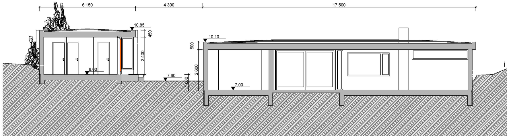
LENGDESNITT HYTTE OG ANNEKS
