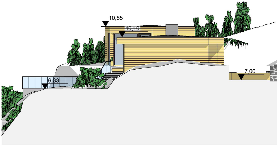
FASADE SØR HYTTE
