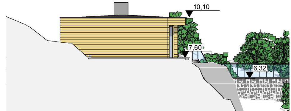
FASADE NORD HYTTE
