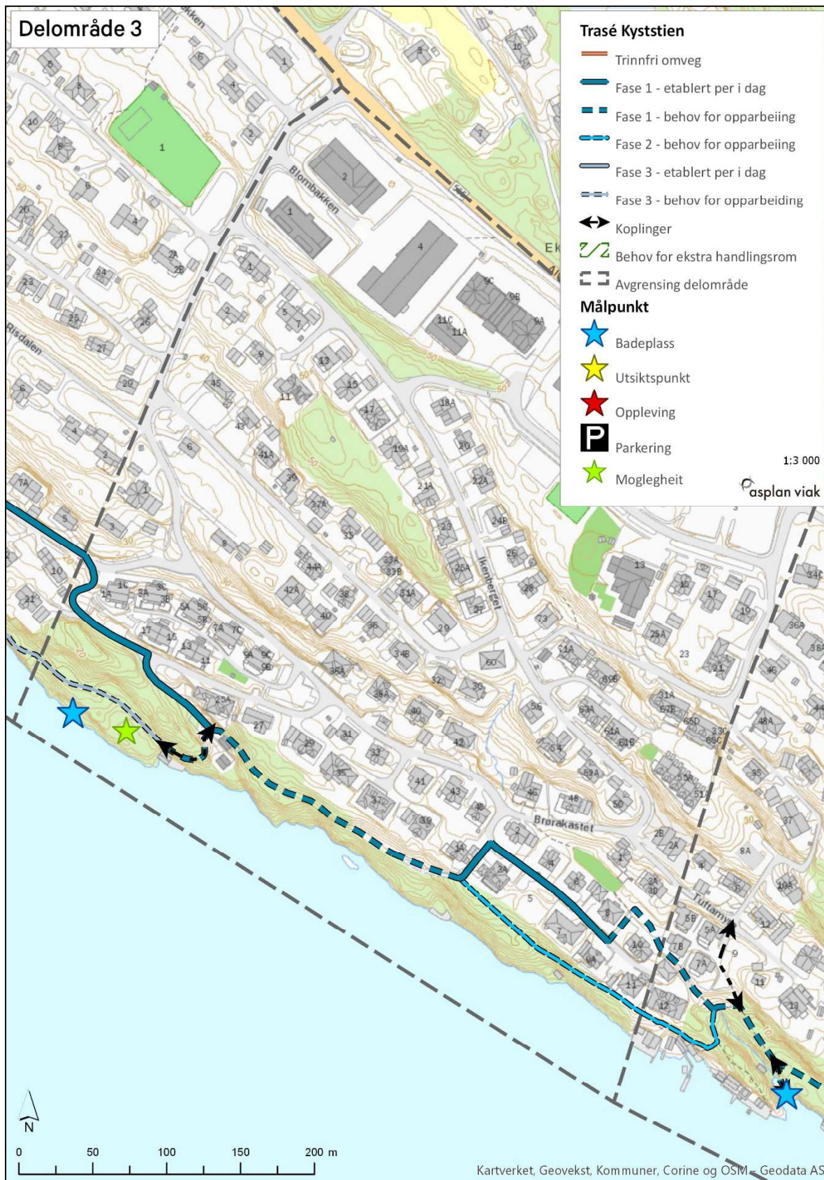
Figur 18: Delstrekning 3 – forslag til trasé.
