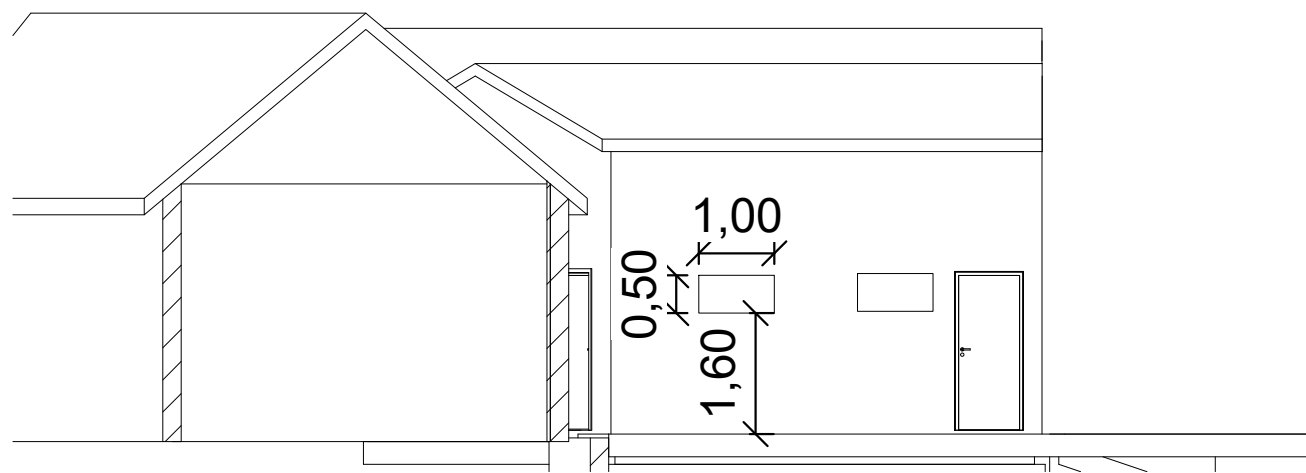
② Section 5 1 : 100
