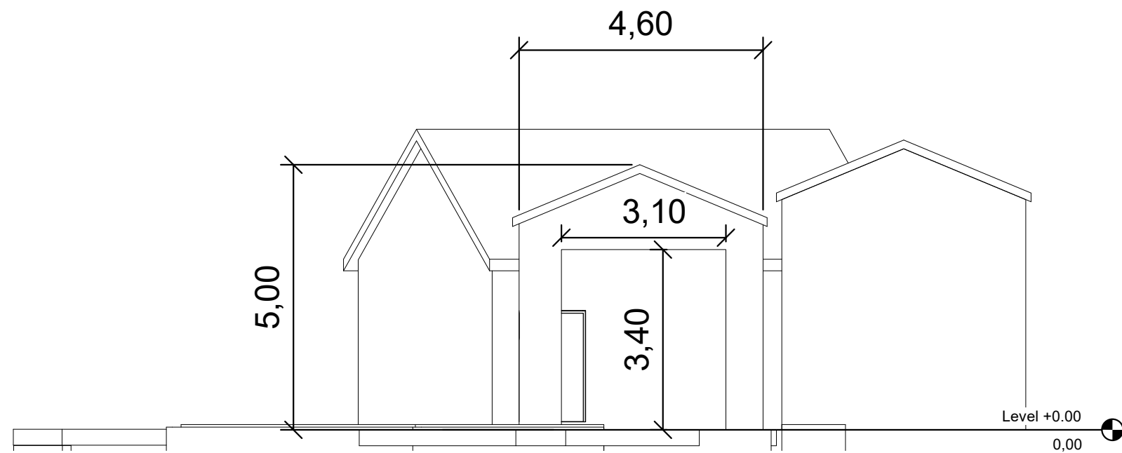
① Section 4 1 : 100
