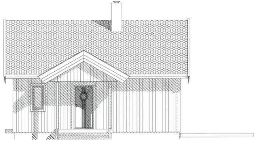
FASADE NORD-ØST
