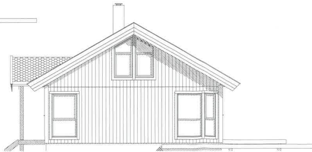
FASADE NORD-VEST
