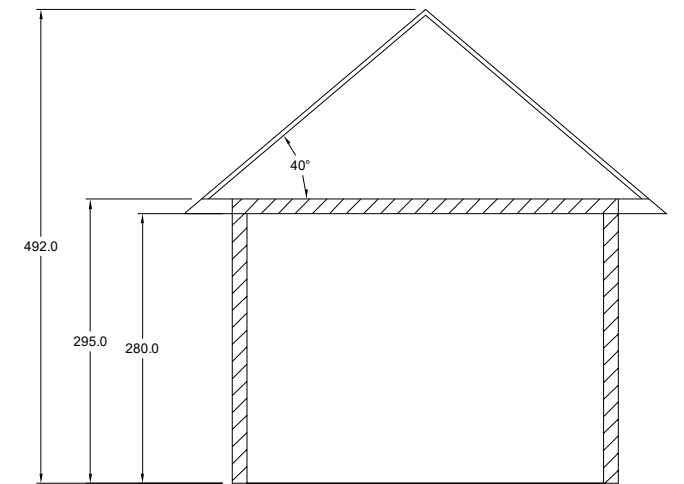
SNITT
