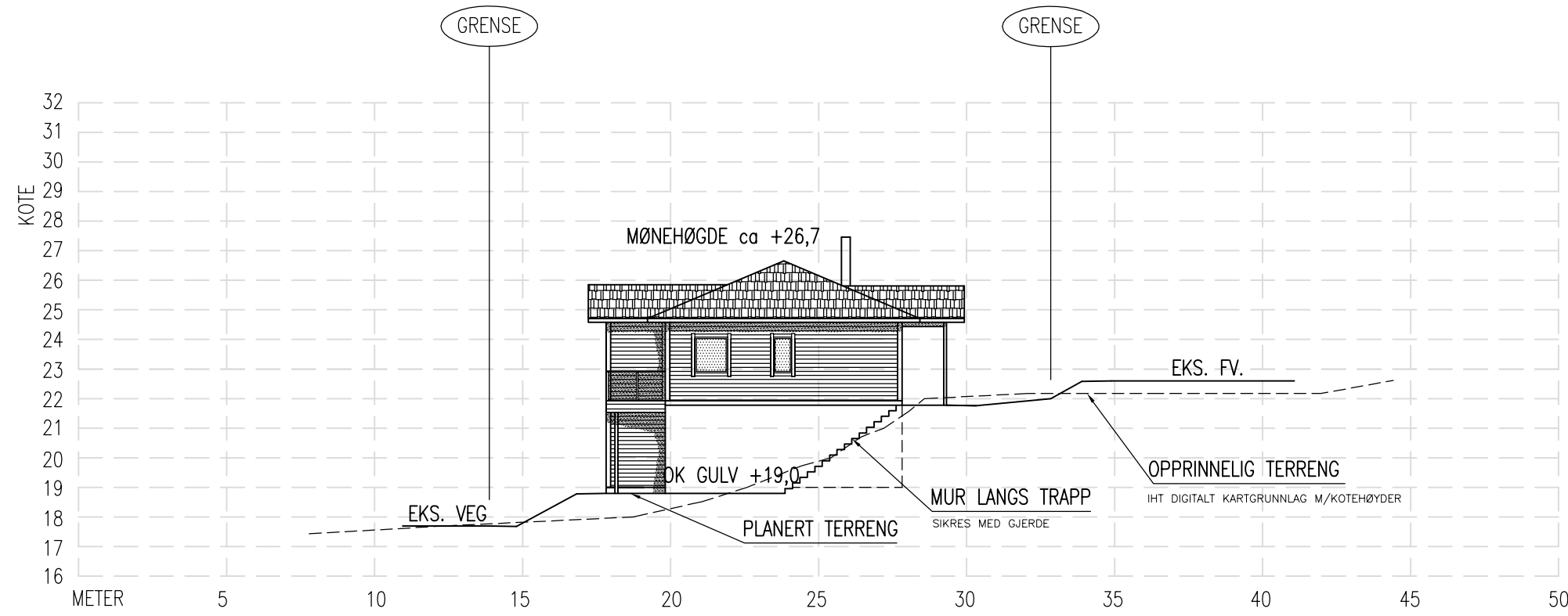
TERRENGPROFIL A-A
