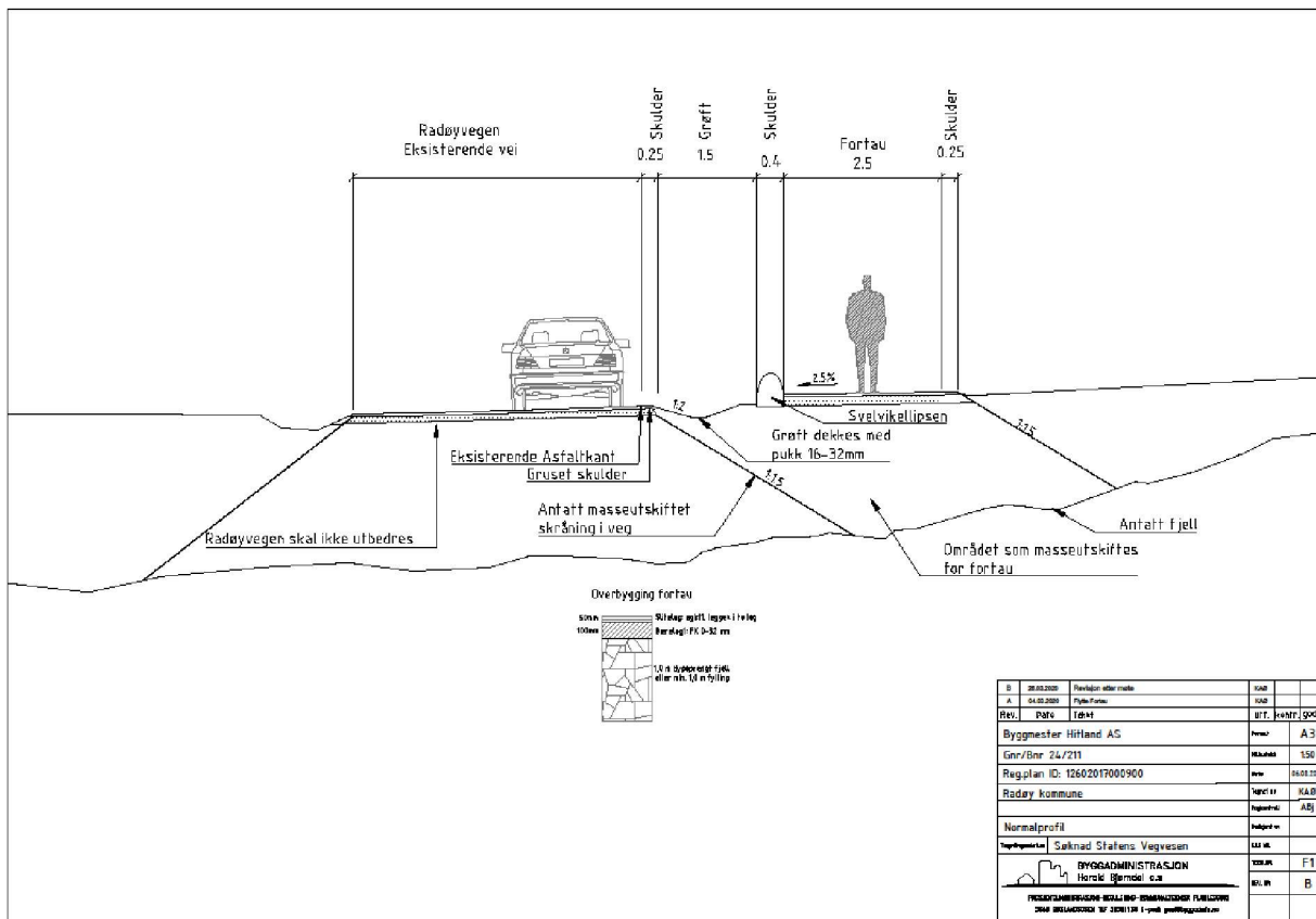
Profiltteikning nytt fortau og grøft
