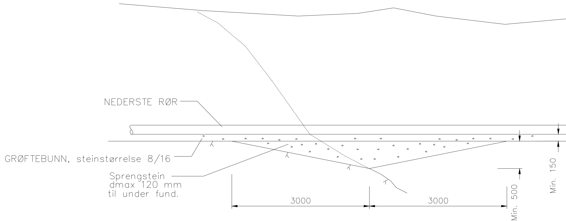
UTKILING AV GRØFTEBUNN VED OVERGANG FJELL/JORD
