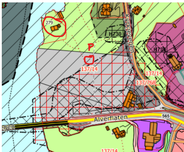
Fig: KDP Knarvik - Alversund med Alverstraumen. Fritidsbustad er vist som LNF - føremål, medan parkering (P) er vist som trafikkareal i samband med regulering av ny Alversund bru.
