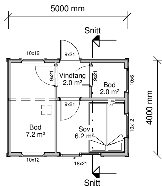
ETASJE 1
