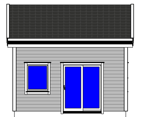
FASADE SØR
