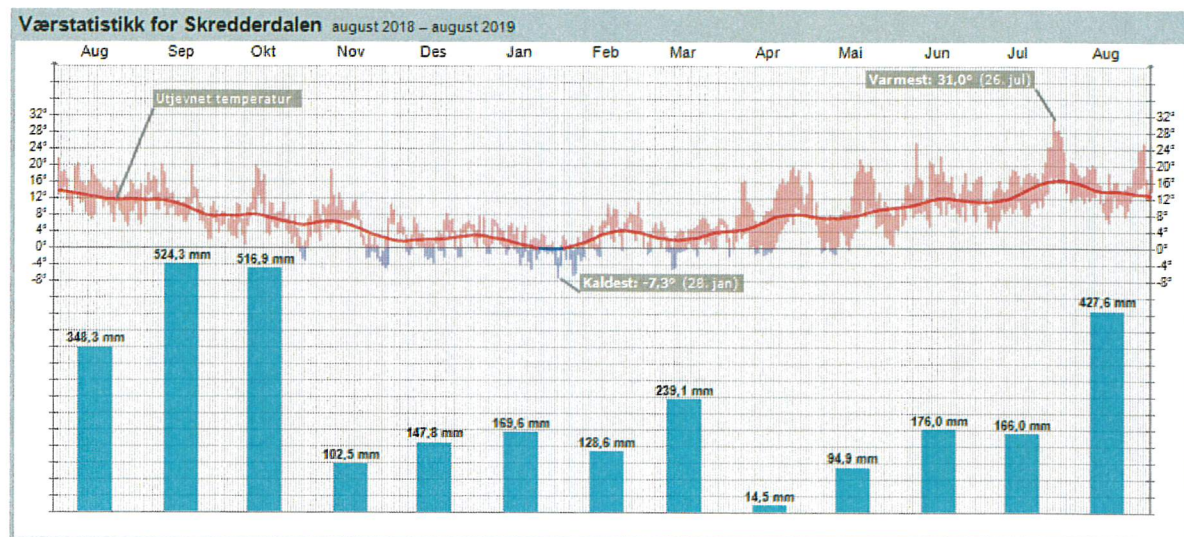
Figur 2-7. Værstatistikk for Skredderdalen målestasjon
