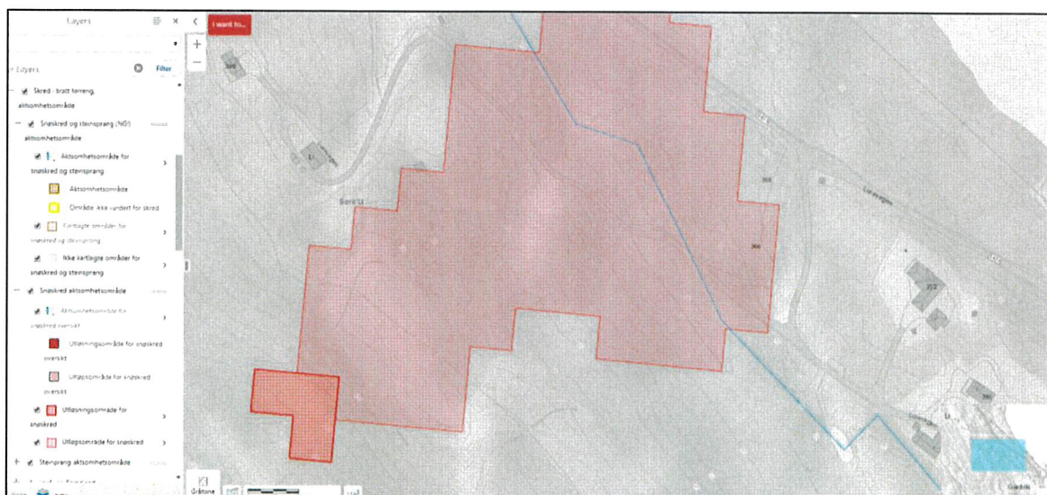
Figur 2-6. Aktsomhetskart for snøskred fra NGU/NVE.
