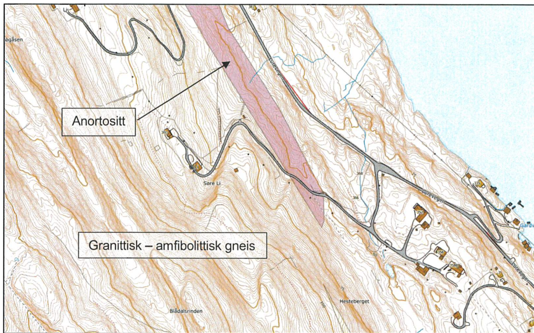
Figur 2-4. Bergrunnsgeologisk kart over planområdet og omgivelsene.
