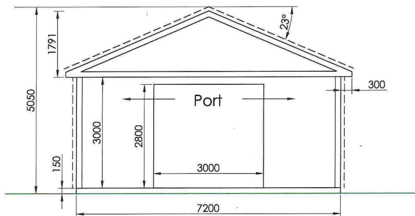
SNITT
