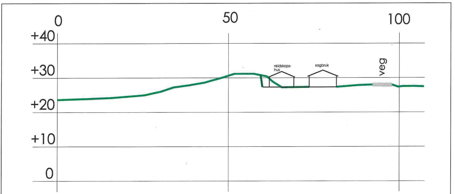
Gbnr. 24/13 Harald Mellingen Reidskaps-hus ved sagbruk Snittplan og terrengsnitt utkast 090318 / VM
