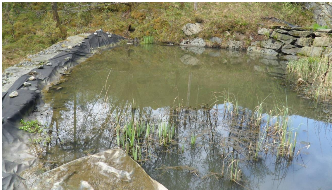
Den øvre dammen har overløp i toppen av dammen.
