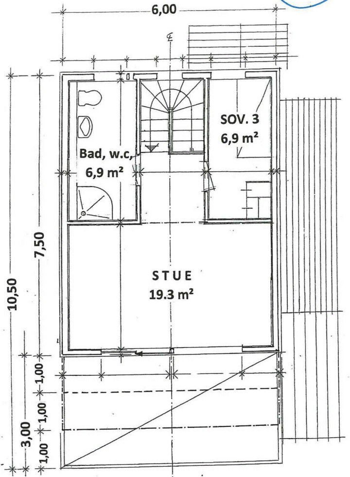
PLAN 2. etasje
