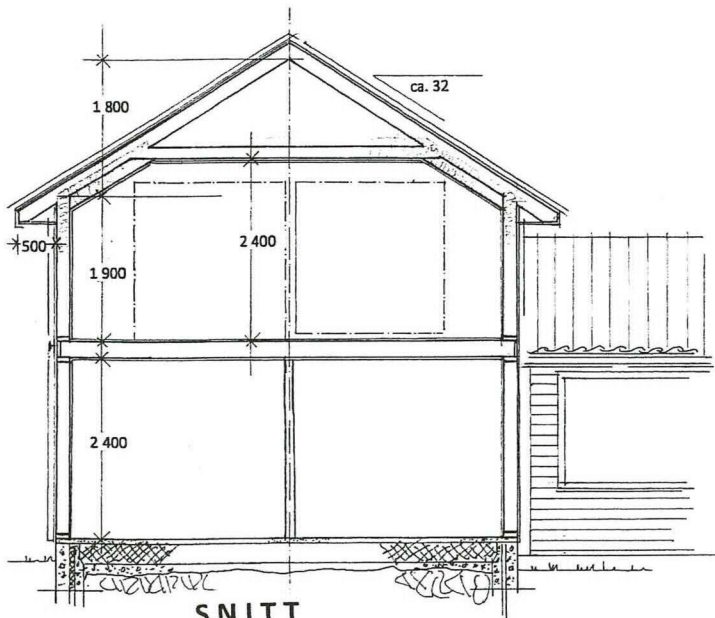
SNITT
