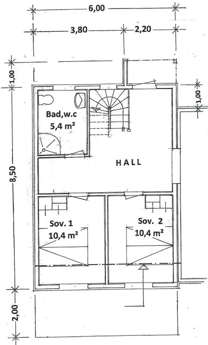
PLAN 1. etasje
