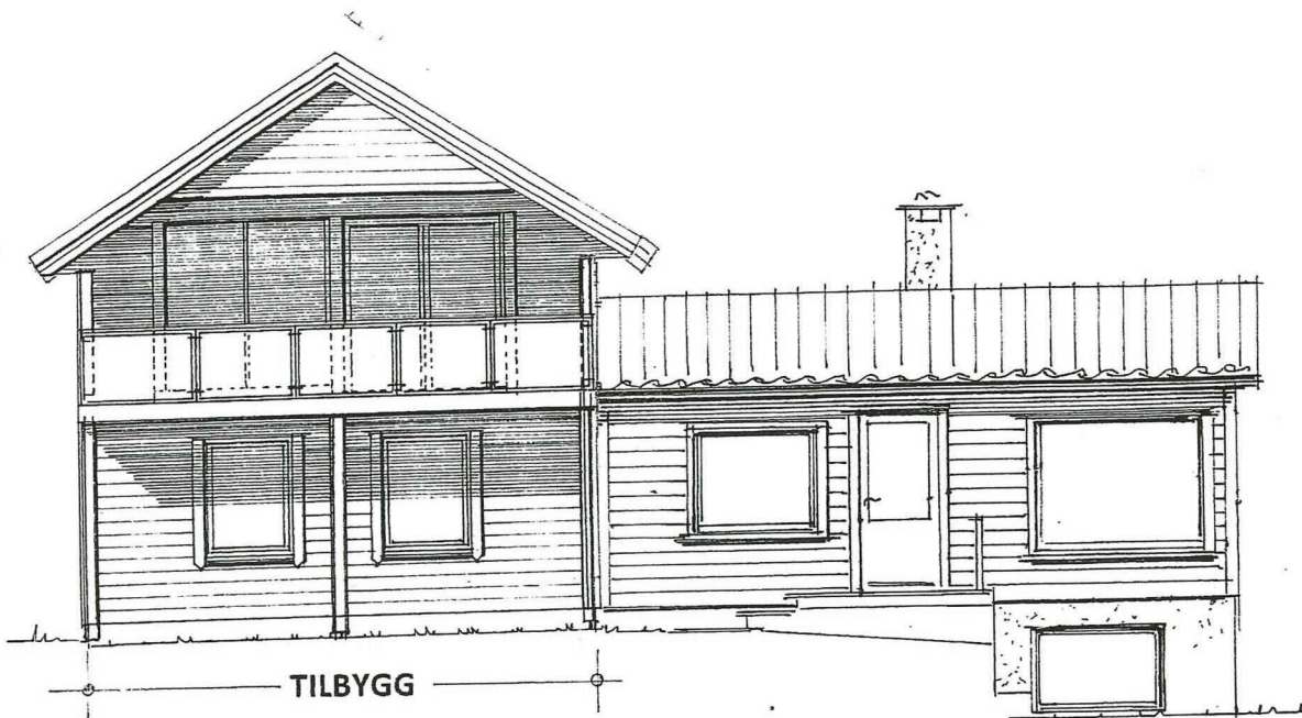
Fasade mot SØR-VEST
