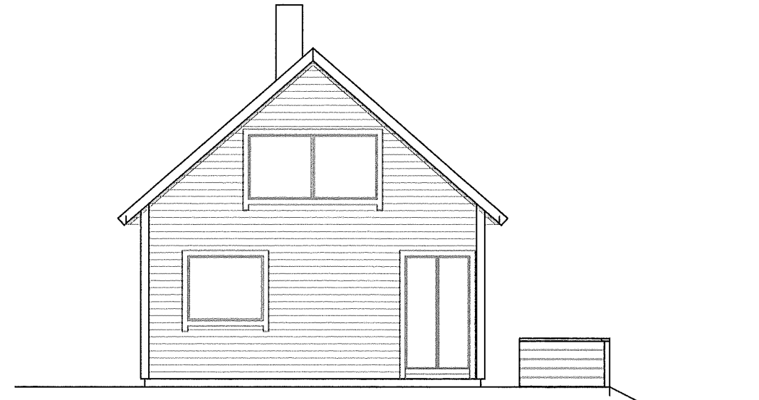
FASADE MOT NORD-VEST
