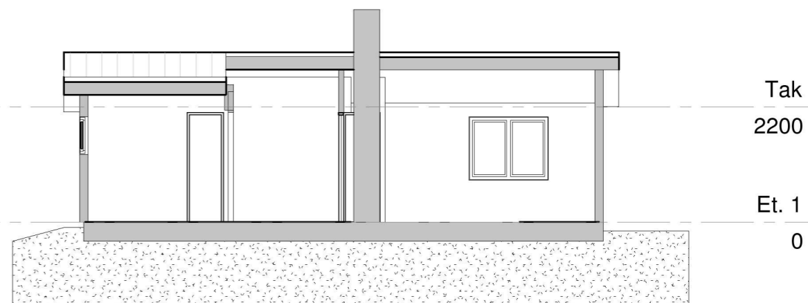
Snitt B - B EKS 1 : 100
