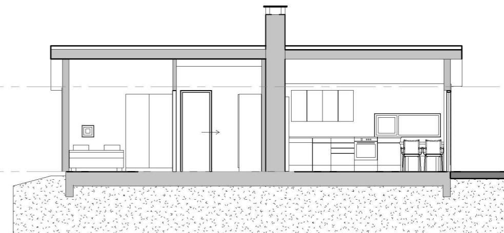
Snitt B - B 1 : 100
