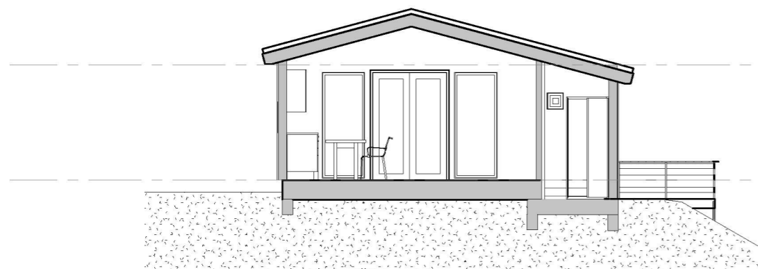
Snitt A - A 1 : 100
