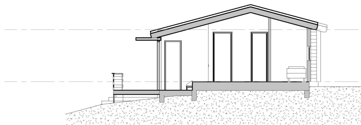
Snitt C - C 1 : 100
