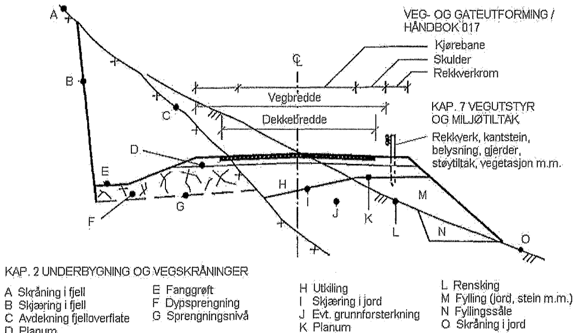
Figur 1: Normalprofil fra 017
