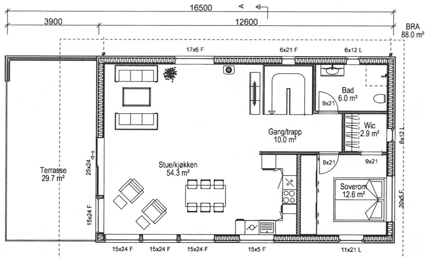
PLAN 1 ETG.
