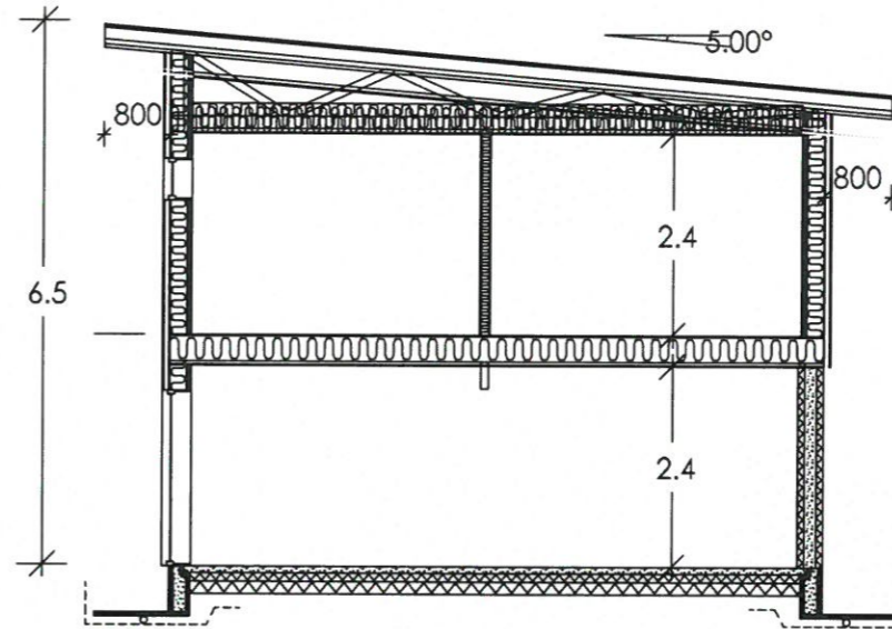
SNITT A-A
