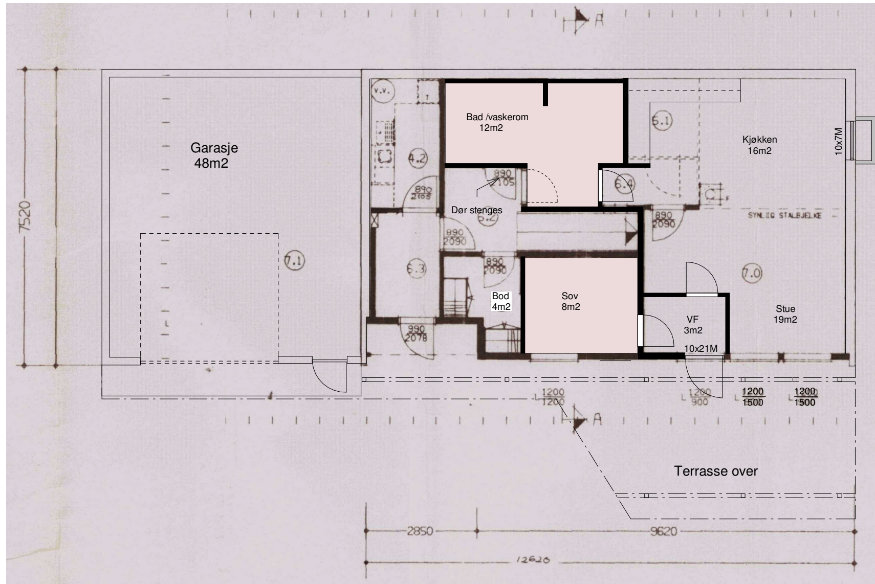
Plan underetasje
