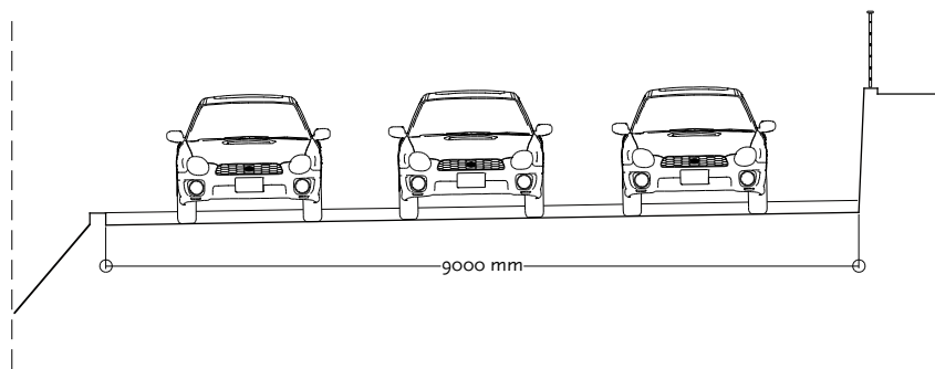
SNITT B - B
