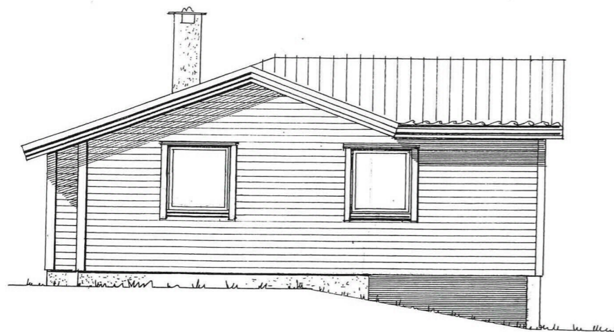
Fasade mot SYD-ØST
