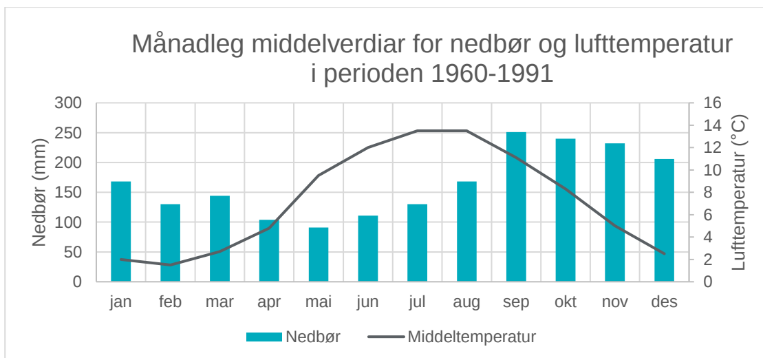
Figur 9. Normalverdiar for temperatur og nedbør registret på målestasjon Radøy-Manger (Strn. 52500).
