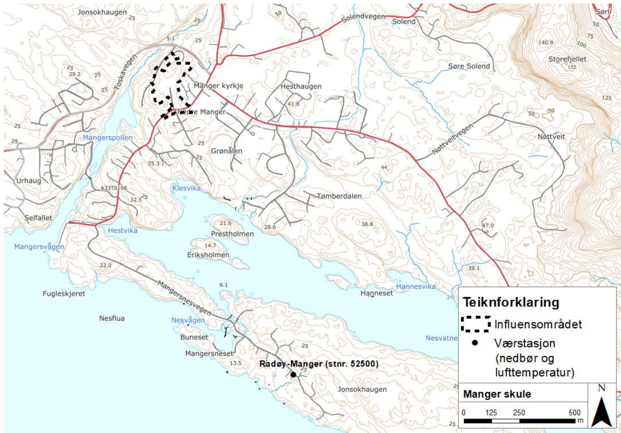
Figur 8. Vêrstasjon ligg sør-søraust for Manger skule.
