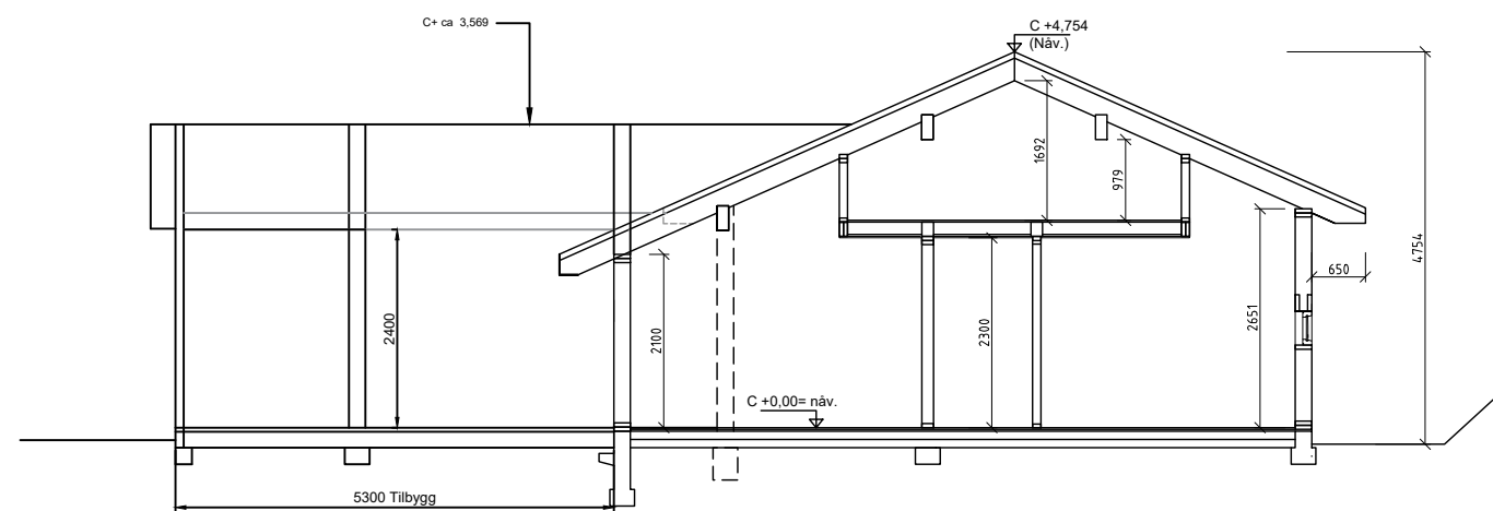
Snitt 1-1
