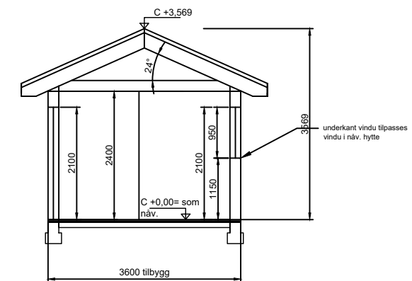
Snitt 2-2
