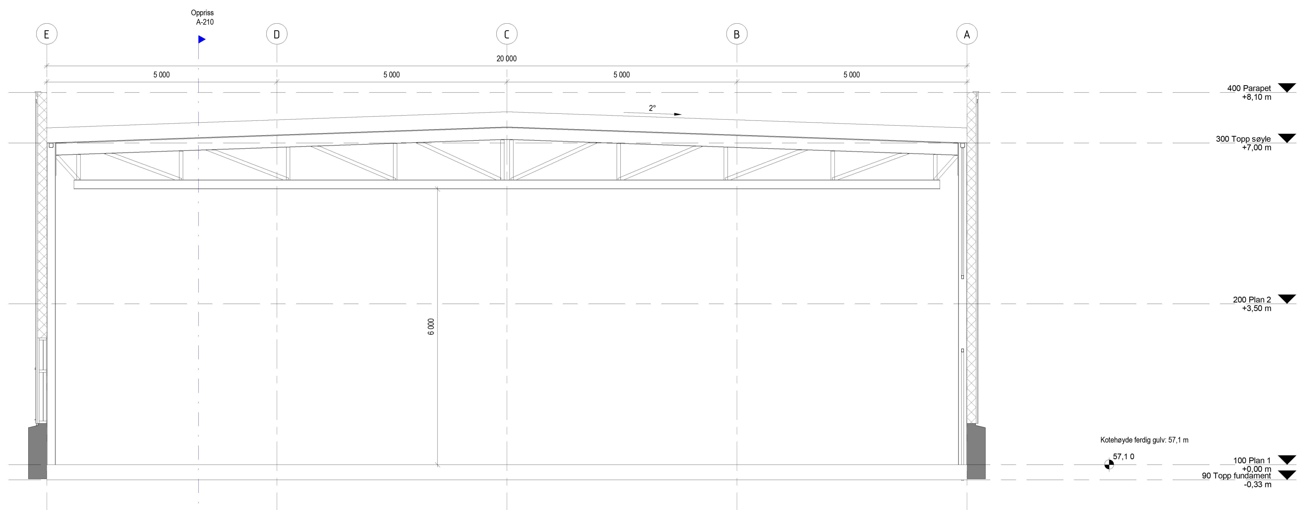
Hovedsnitt 1 : 50
