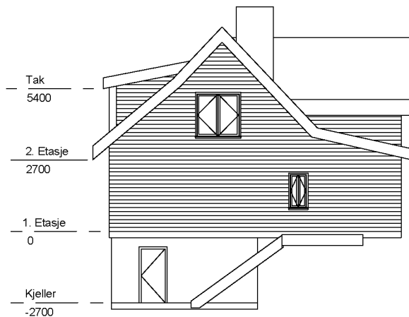
1 Øst 1 : 100
