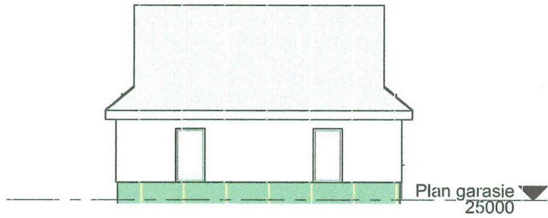
1 Fasade nordvest 1 : 100
