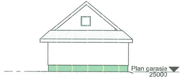
2 Fasade nordøst 1 : 100
