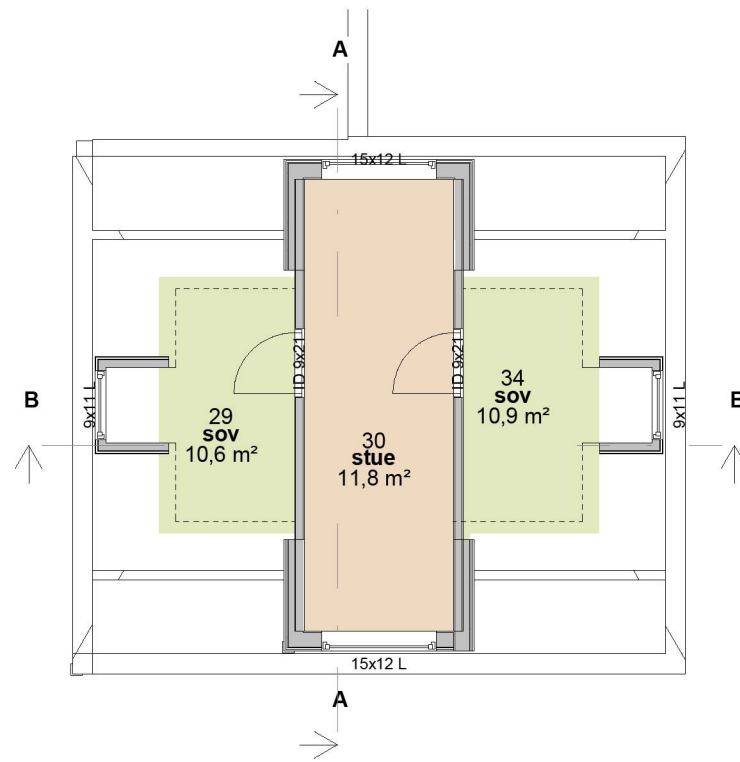
2. Etasje 1 : 100
