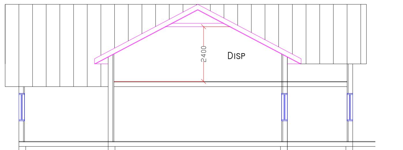
LENGDESNITT
