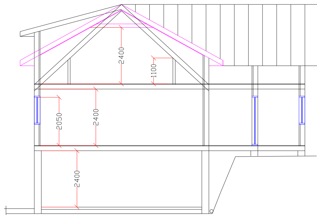
TVERRSNITT
