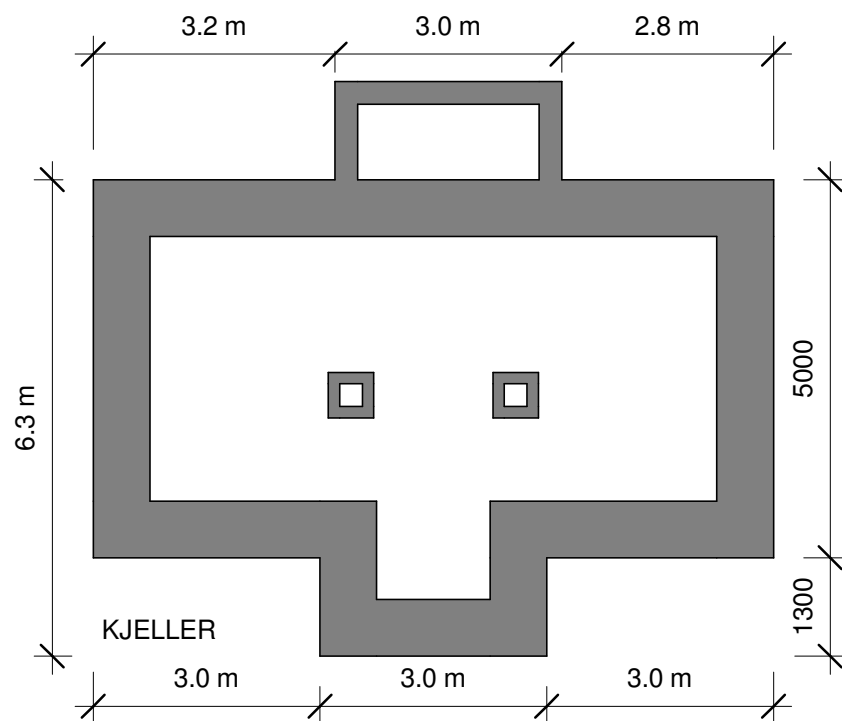
HOVEDPLAN
