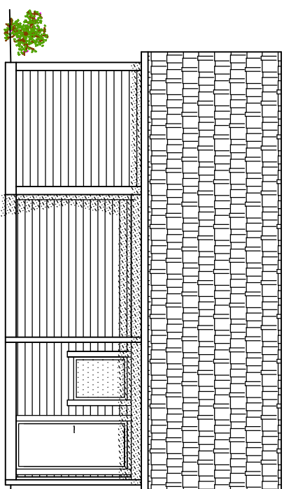
FASADE ØST
