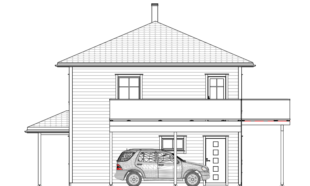
FASADE 2 1 : 100
