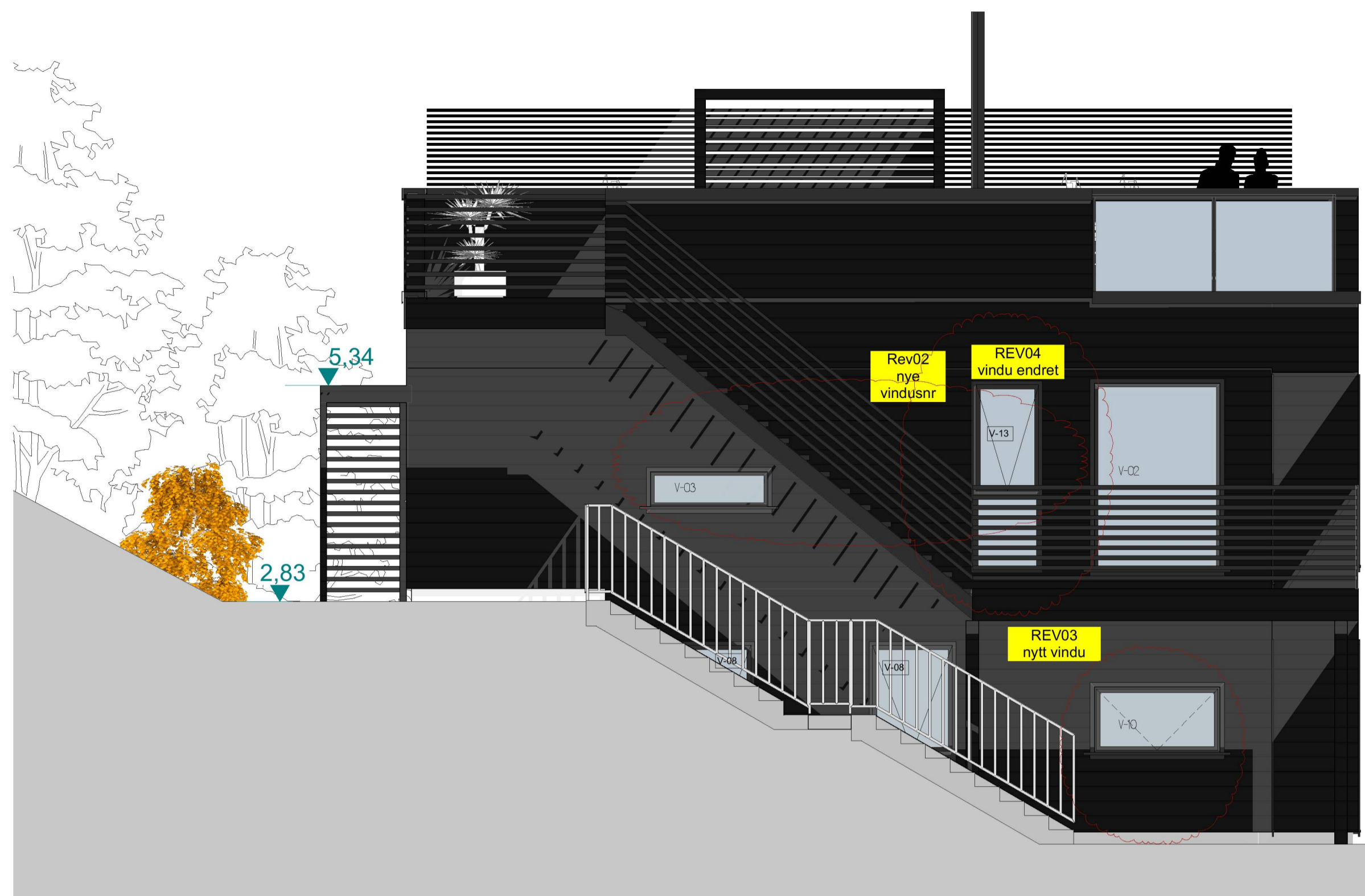
1:50 Fasade 4
