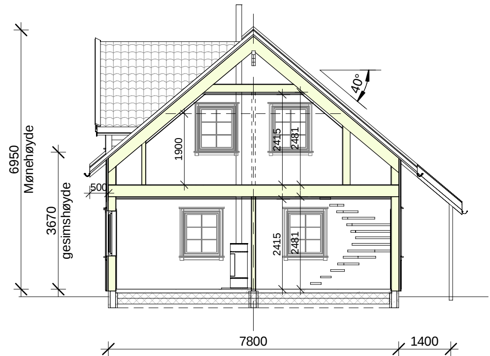
Snitt A-A
