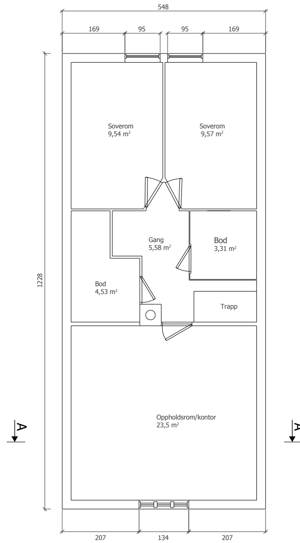
Plan 2. etg.
