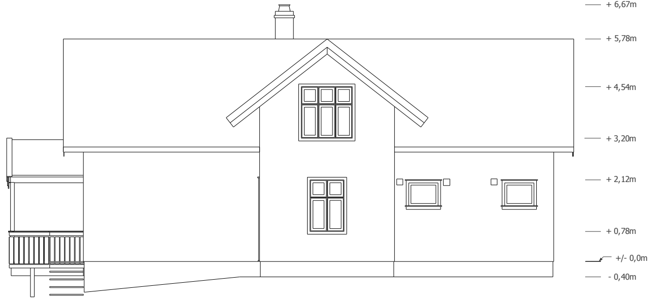
Fasade - øst
