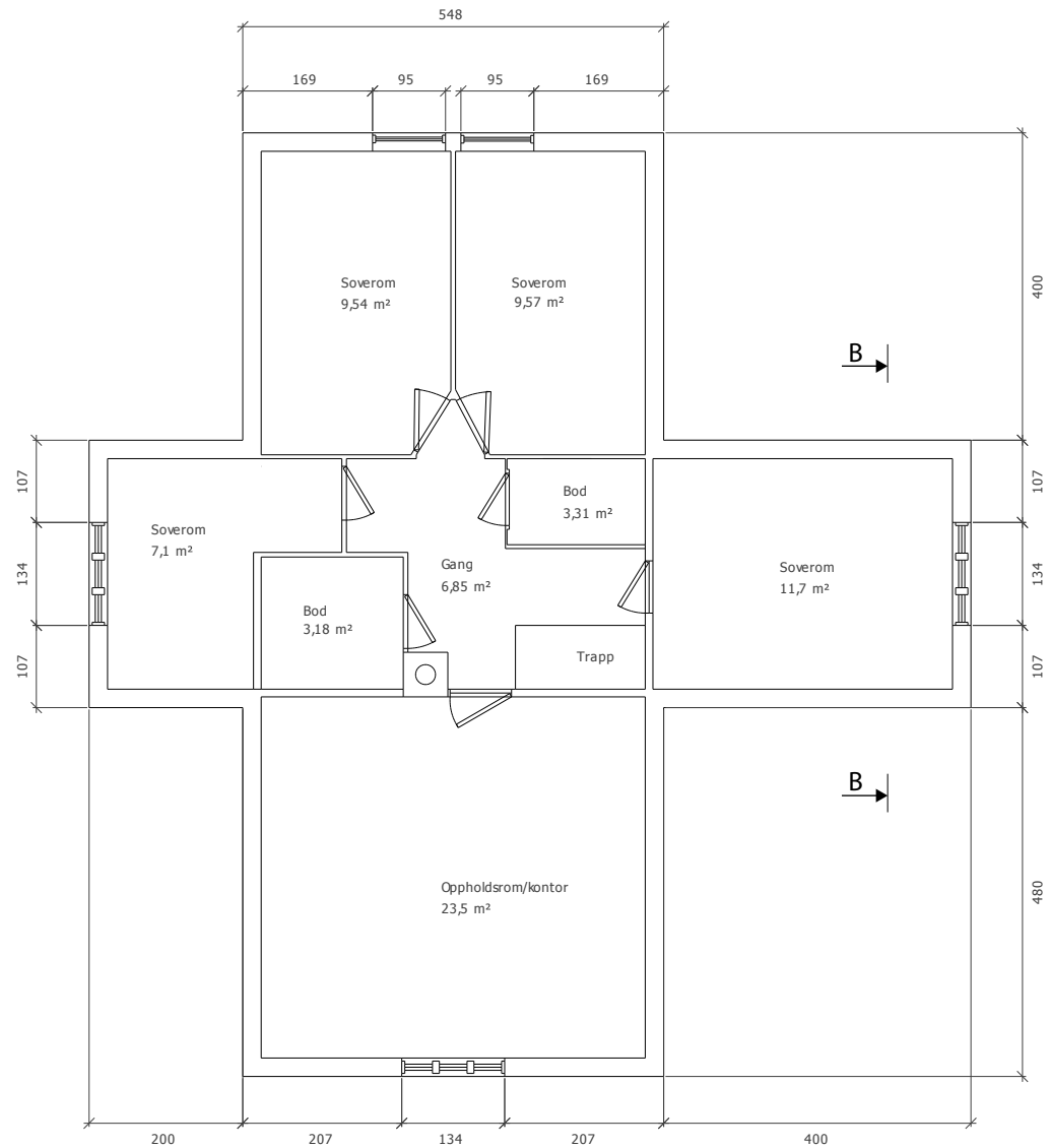
Plan 2. etg.
