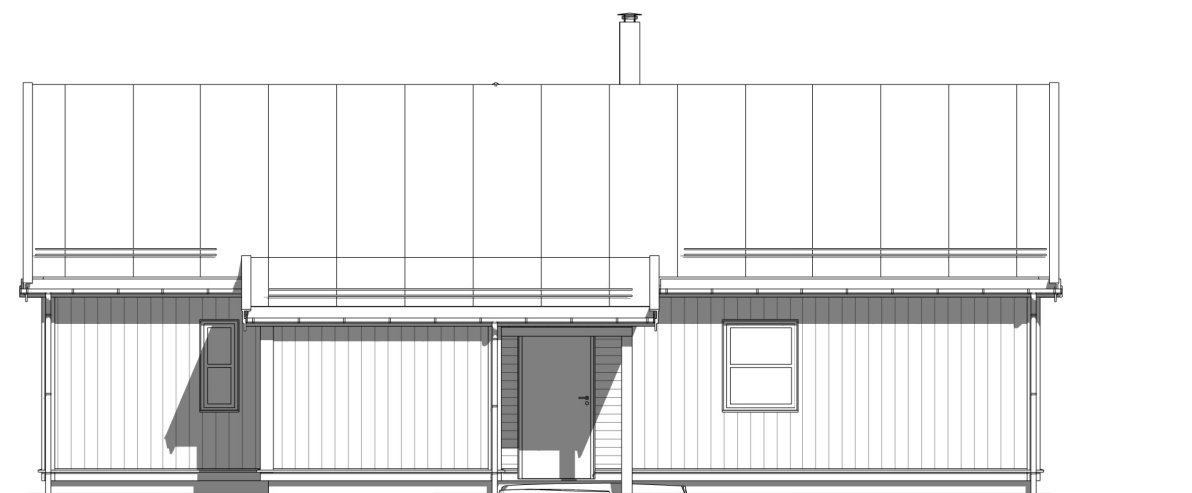
sørvest 1 : 100
