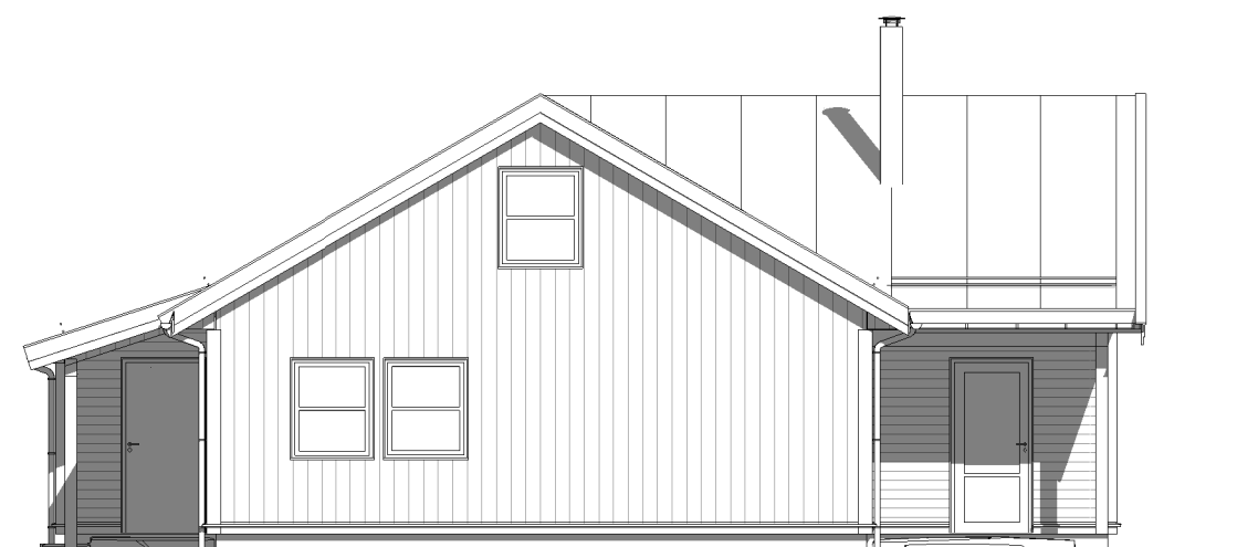
sørøst 1 : 100
