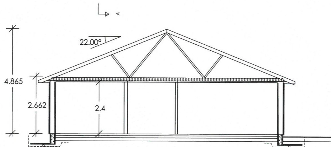
SNITT A-A
