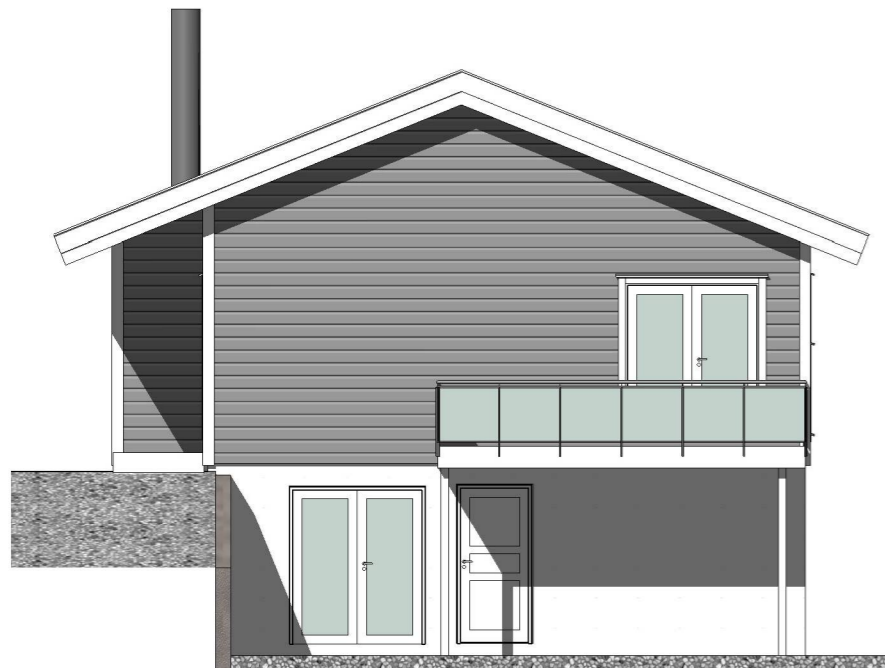
Fasade mot sør-øst 1 : 100
