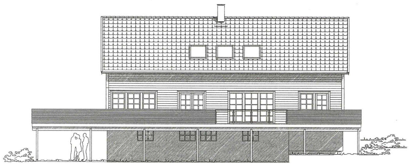
VEST
